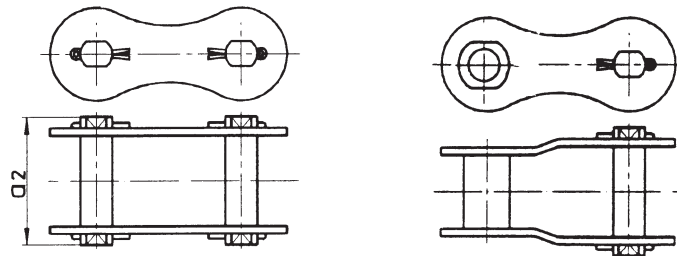
A Steckglied mit Splintverschluss
